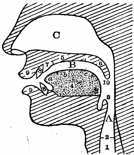
英语发音器官图
