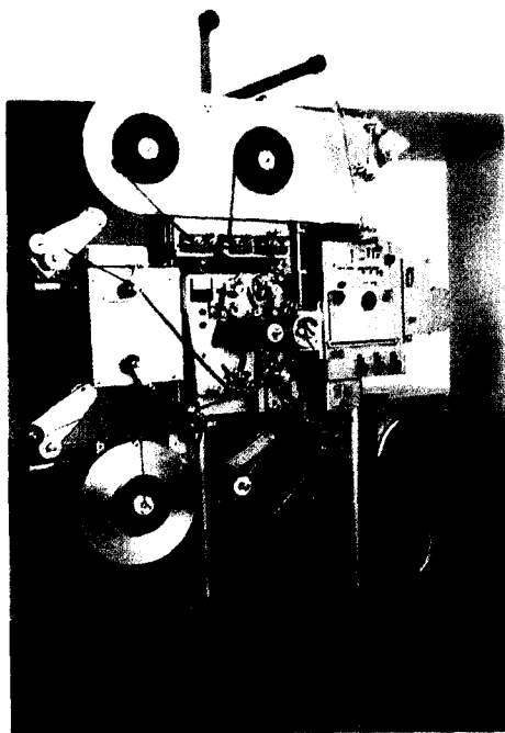
用于洗印电影拷贝的SEIKI加色光缩放机
