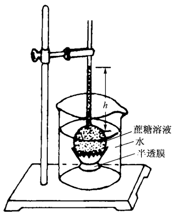
图 1-1 渗透装置
