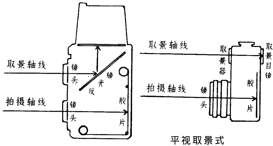
双镜头反光取景式 图 1-2
