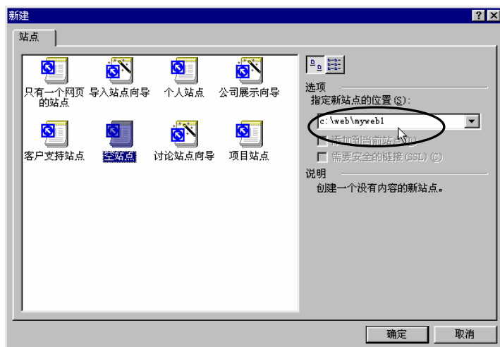
图 1.2 “新建”对话框
