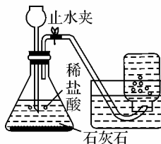
A. 制取 \text{CO}_2
