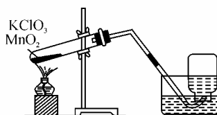
B. 制取 \text{O}_2
