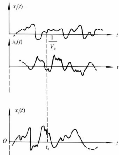
图 1.2 热噪声电压的样本曲线
