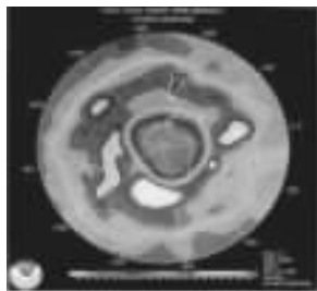
图 2-22 南极臭氧层空洞
