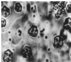
图 2-14 结晶牛胰岛素
