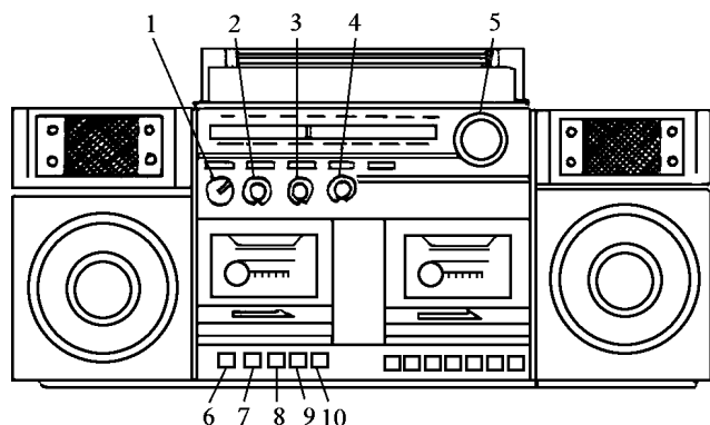
图 1 便携式收录机外观图
