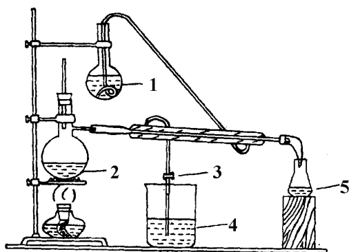
图 11-11 石油蒸馏实验装置
