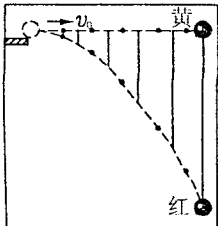
图 1 与自由落体运动的比较 图 2 与匀速直线运动的比较
