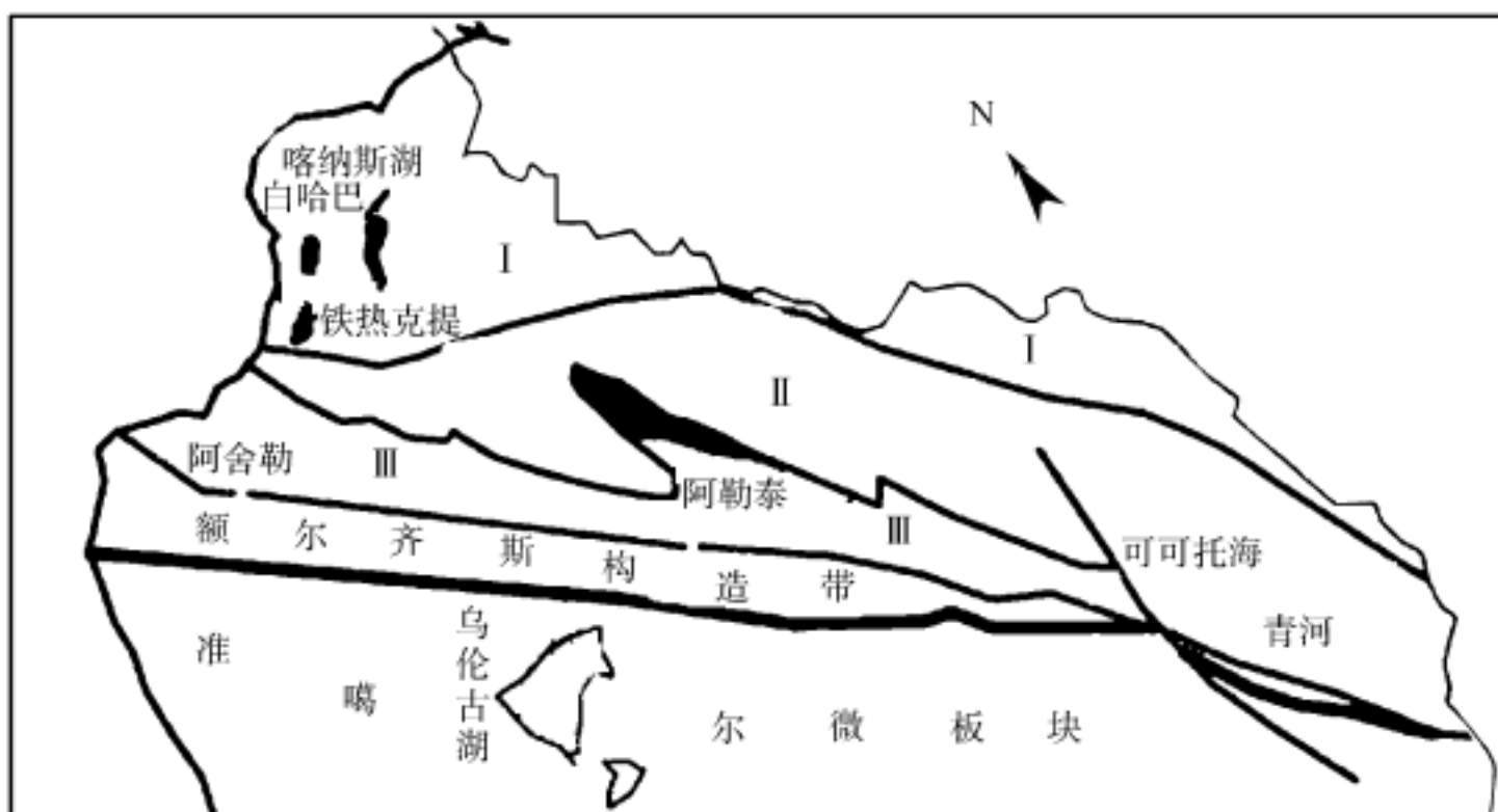
图1 阿尔泰构造分区及上奥陶统分布图
