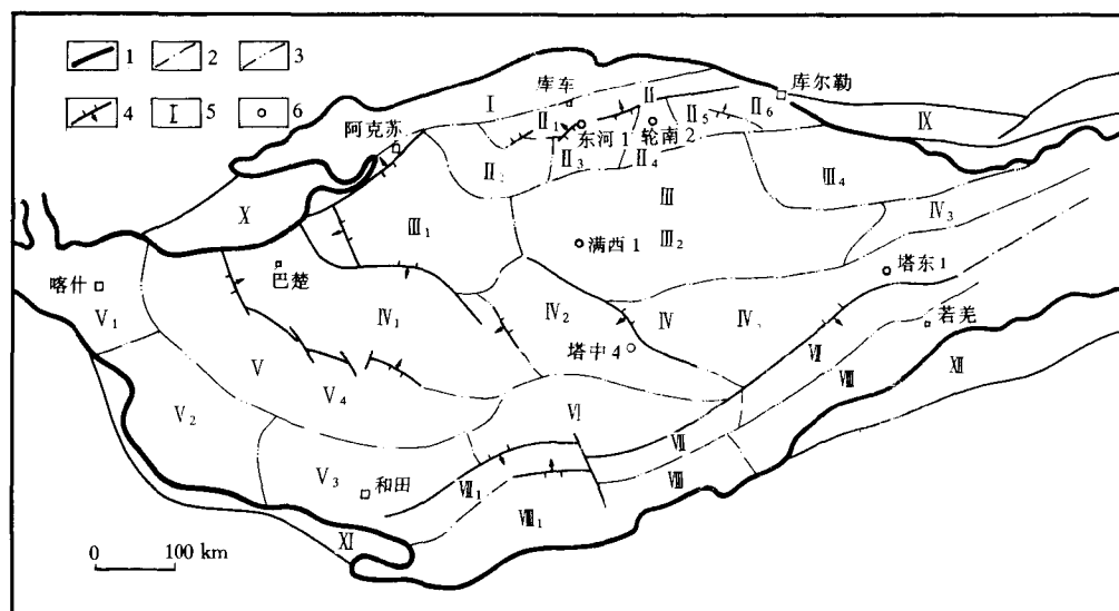
图 1—1—1 塔里木盆地构造区划图
