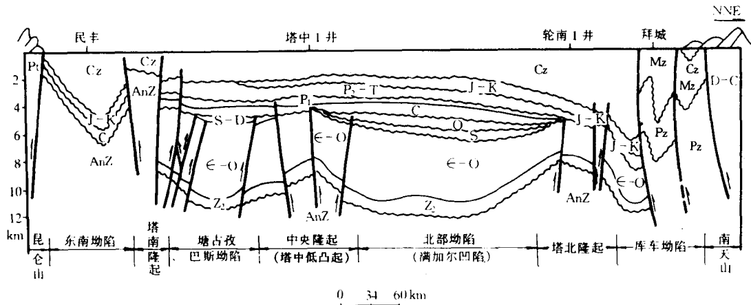
图 1—1—2 塔里木盆地地质构造横剖面
