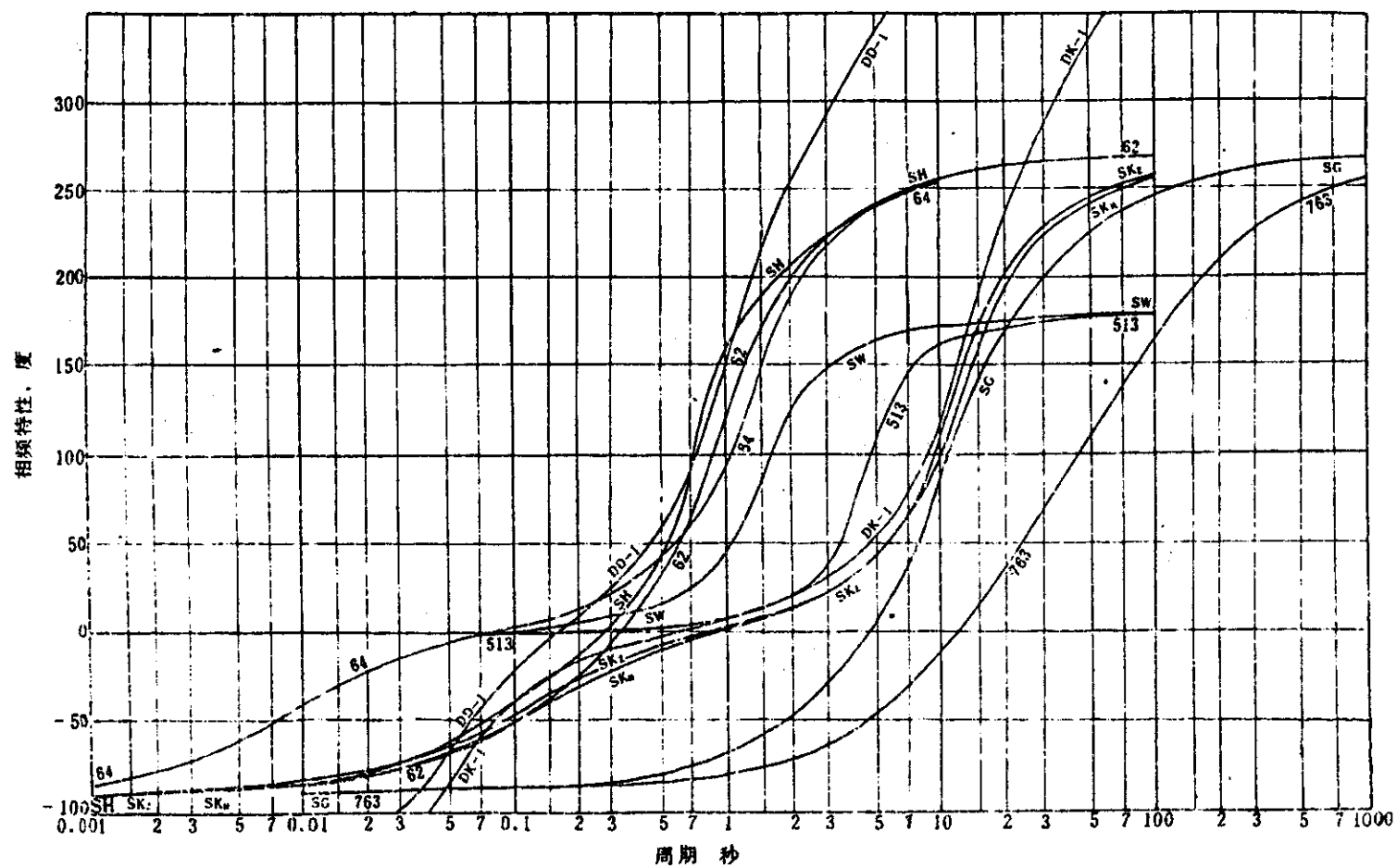
仪器相频特性曲线
