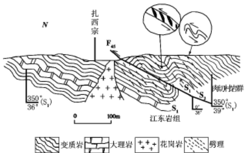
图 1 - 10 扎西宗断层构造剖面示意图
