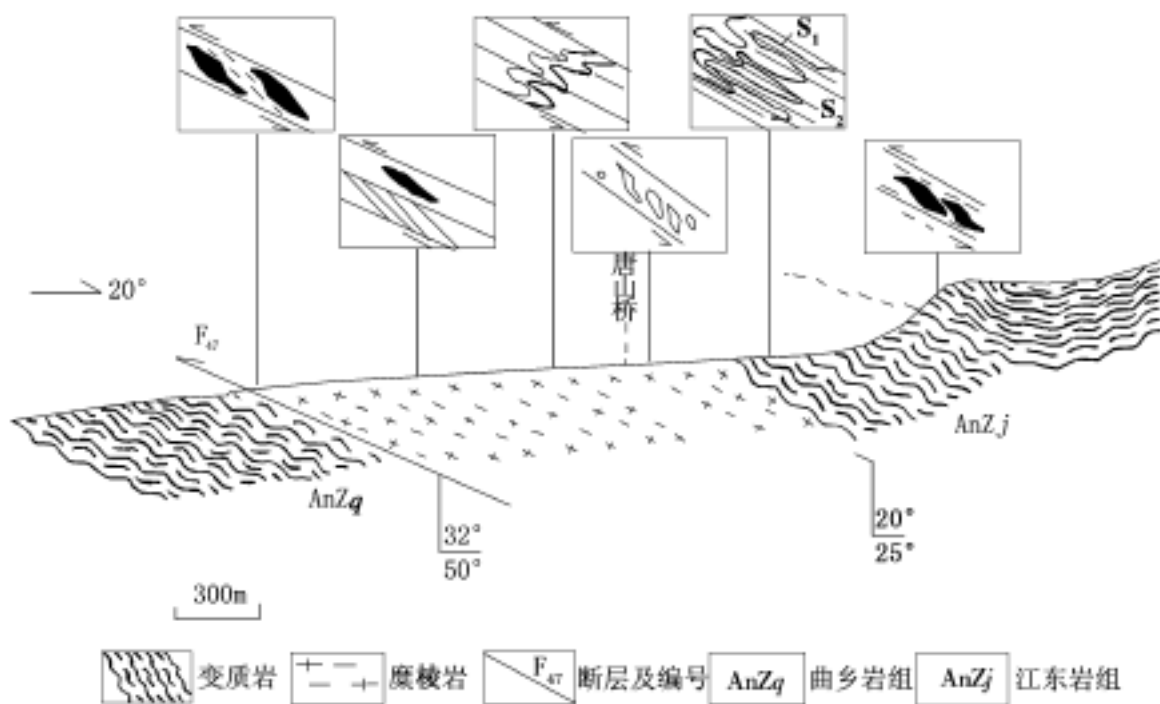
图 1 - 11 康山桥韧性剪切断层带构造剖面示意图
