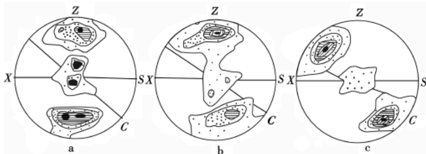
图 1 - 5 糜棱岩石英 C 轴组构图（XZ 切面，下半球投影）
