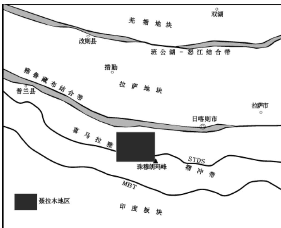
图 1 - 1 大地构造略图
