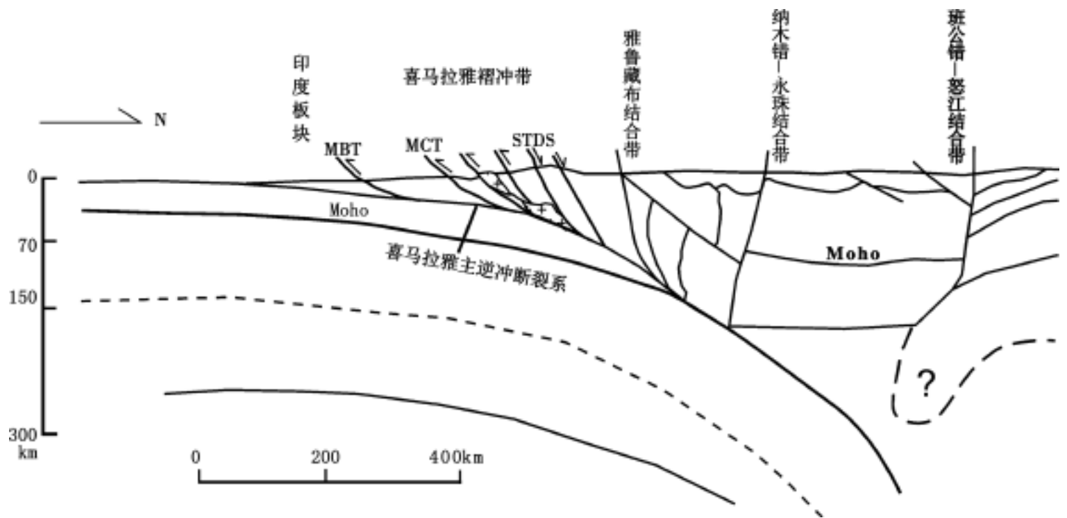
图 1 - 2 印度板块与欧亚板块碰撞构造模式图
