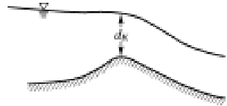
图 1-10 低水断面控制示意图
