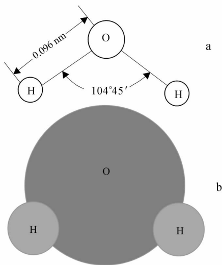
图 1-1-1 水分子中氢氧原子核的空间排布
