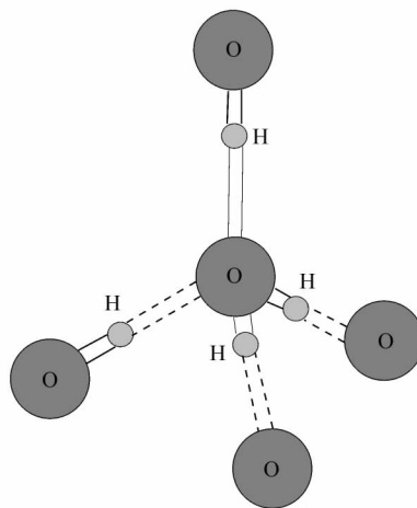
图 1-1-5 相邻冰分子间的四面体构形
