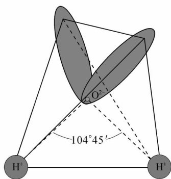
图 1-1-3 水分子的几何外形
