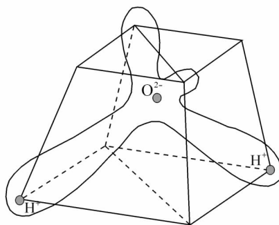
图 1-1-4 水分子核外电子云外形
