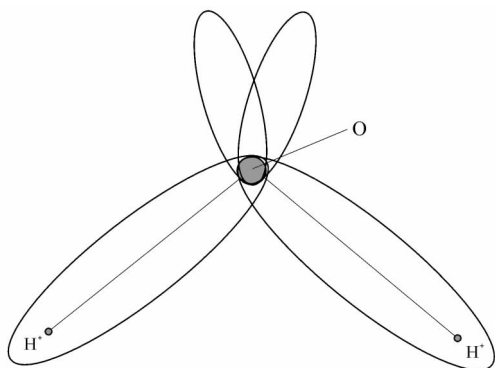
图 1-1-2 水分子核外电子轨道示意图 联接。
