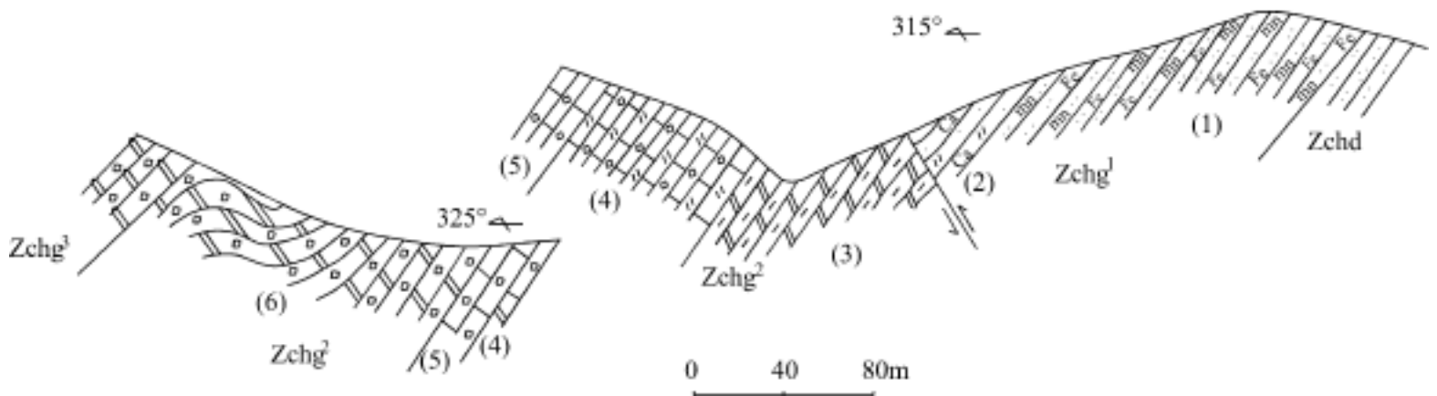
图 2-3 建平化石里沟梁高于庄组一、二段剖面图
