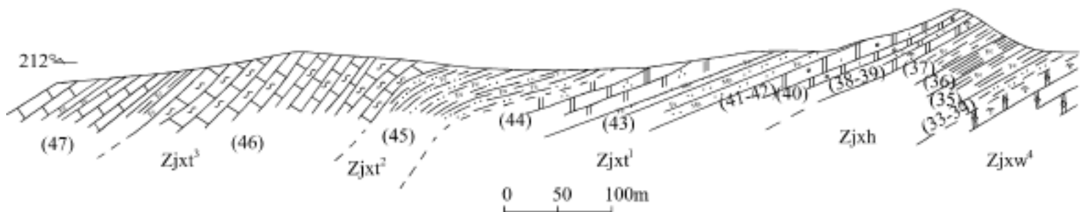
图 2-6 喀左县中三家乡石灰窑子—轱辘井剖面
