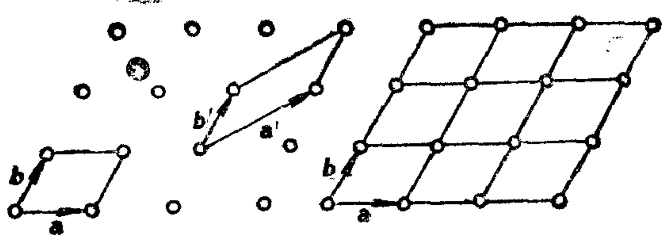
图1-2 平面点阵与平面格子(面网)
