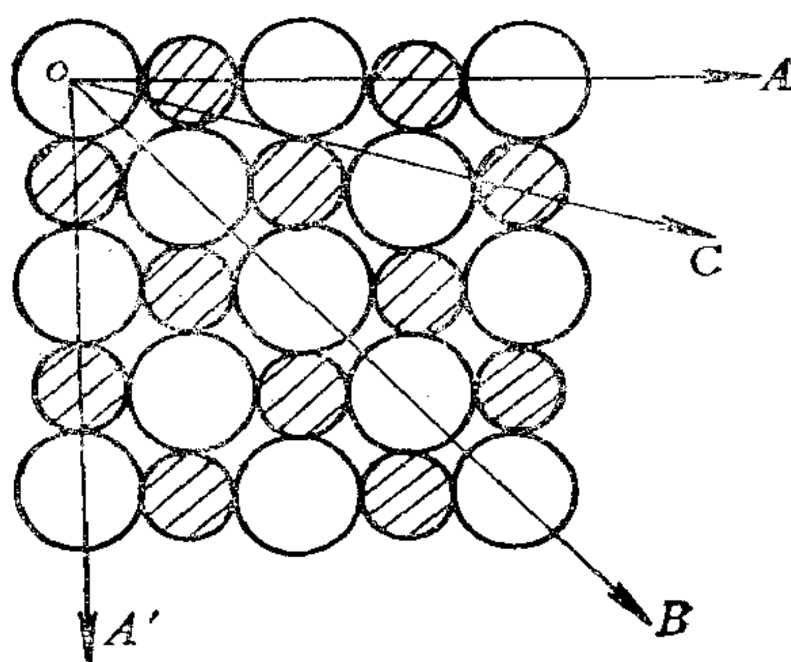
图1-5 晶体的均匀性、各向异性及对称性之示意图(图中画出NaCl晶体结构中的一个晶面，大圆为Cl - ，小圆为Na + )
