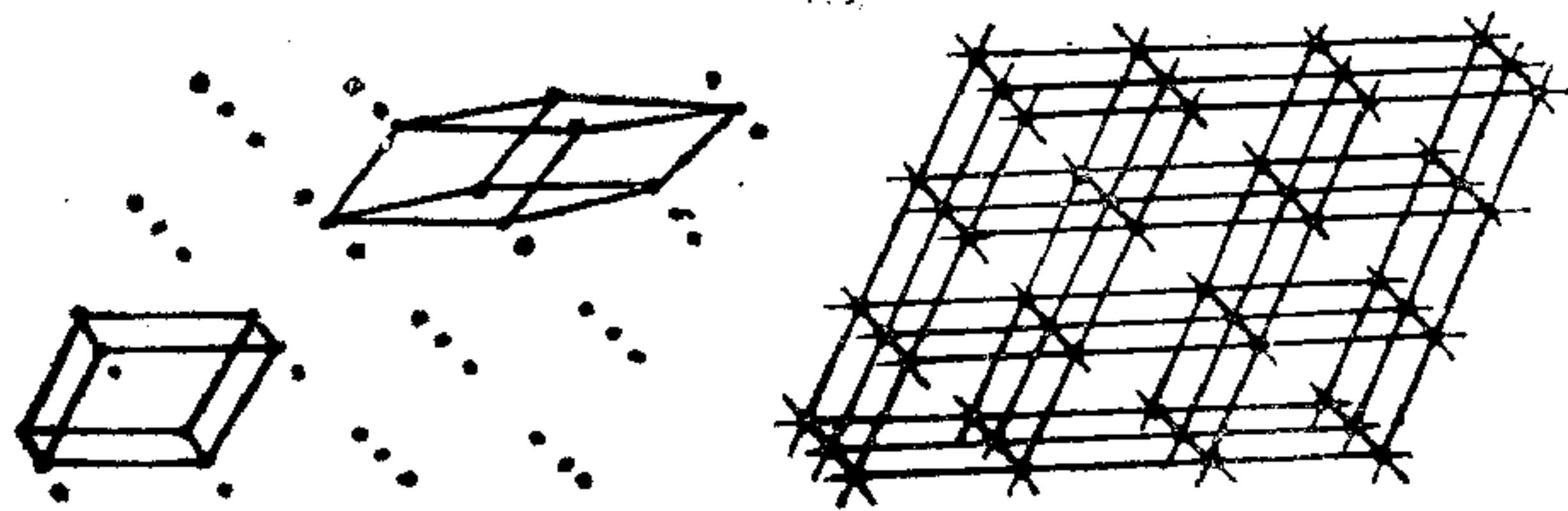
图1-3 空间点阵与空间格子
