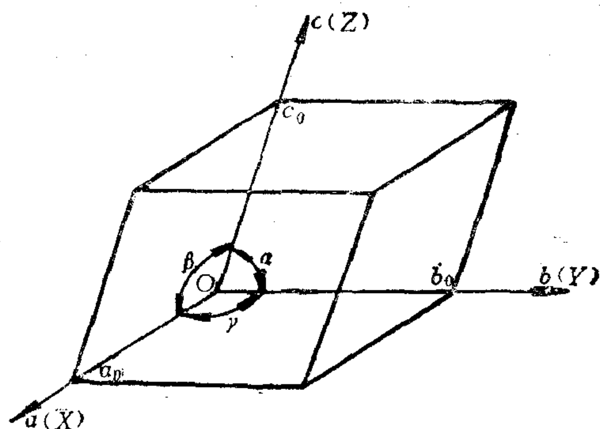
图1-4 晶胞常数
