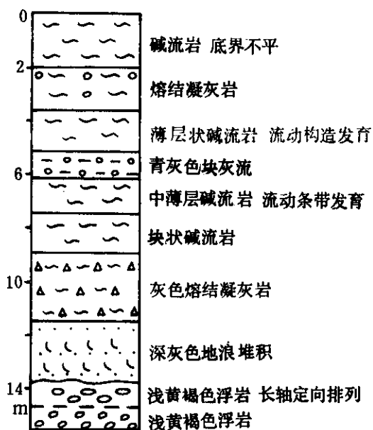
图3 气象站碱流岩质—熔结凝灰岩柱状图
