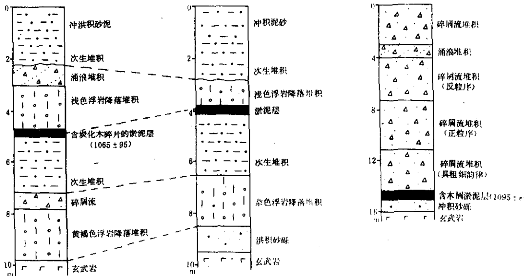
图2 双目峰—圆池—三道白河钻孔柱状图
