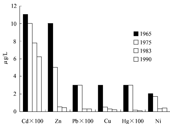
图 10-10 历史上测得海水中痕量元素的浓度 [20]
