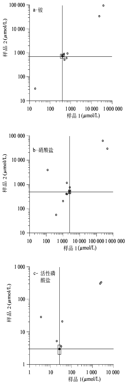
图 15.1 国际政府间海洋委员会西太平洋分会 (政府间海洋学委员会) 1985 年营养盐互校的结果。其中 氨, 硝酸盐以及 活性磷酸盐。图中的实线表明标样的推荐浓度, 方框表示可接受的浓度范围, 而小圆圈代表不同实验室的数据点。
