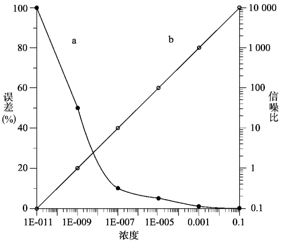
图 猿猿 随元素浓度的改变，测定误差（猿）与测定信噪比（遭）的变化
