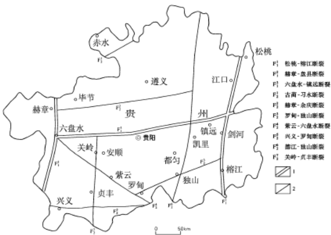
图 12 贵州深部构造略图 1— 一级断裂; 2— 二级断裂
