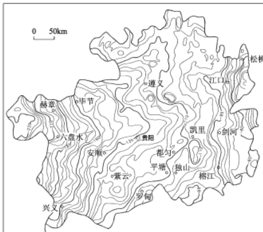
图 11 贵州省布格重力异常平面图(单位: m/s^2 ) (据范发祥, 1999)
