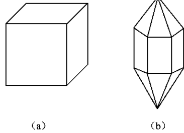
图 圆 圆 矿物的晶形 (a) 圆 圆 硅酸盐晶体 (b) 圆 圆 石英晶体
