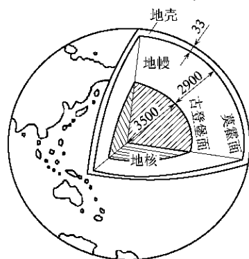
图 1-1 地球内部圈层构造( \text{km} )
