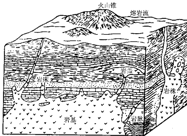
图 圆源 岩浆岩体的产状
