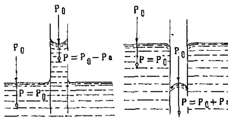
图1-3 毛细现象
