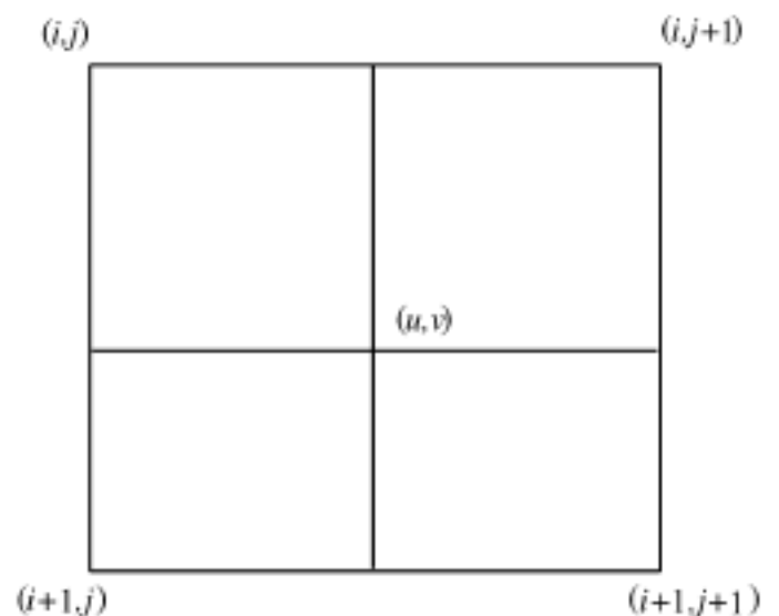
图 1 1 双线性内插法示意图
