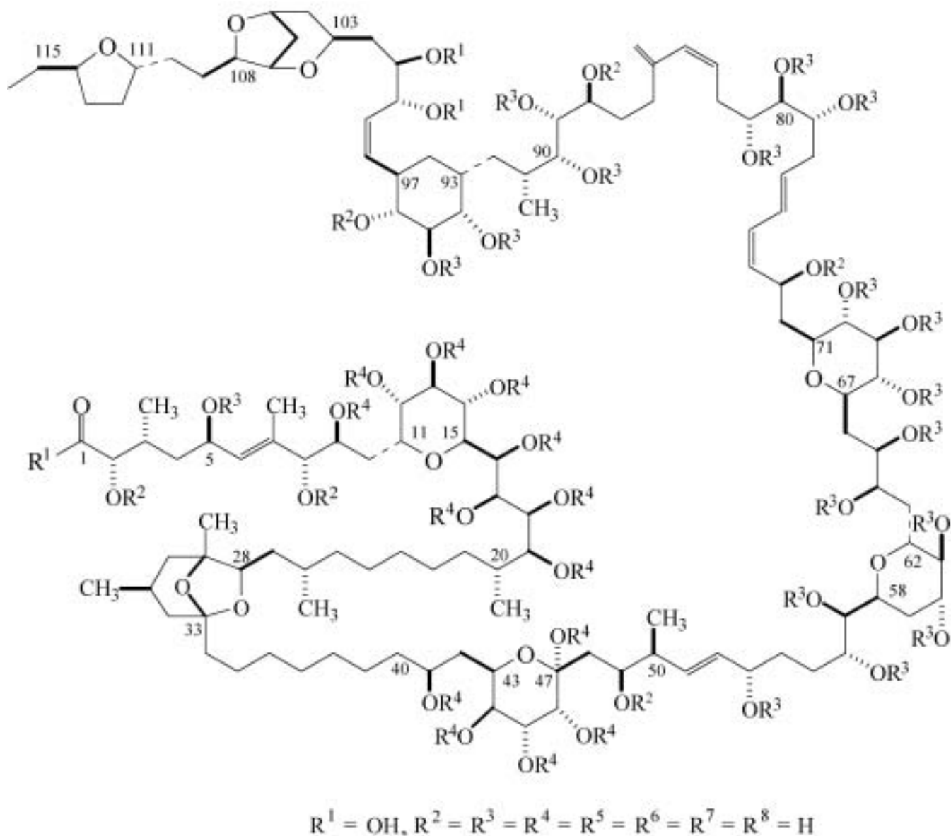
海葵毒素
