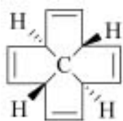
十字四烯的结构
