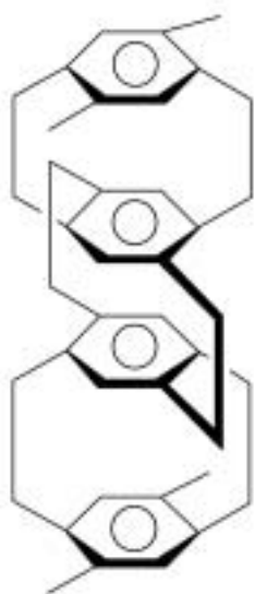
1,2,7,8-二苯并[2,2]-对二蕃烷
