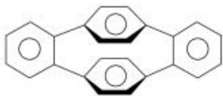
1,2,7,8-二苯并[2,2]-对二蕃烷
