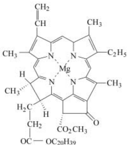
叶绿素的结构
