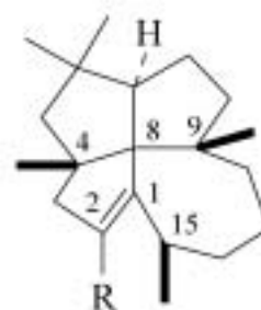
二萜
