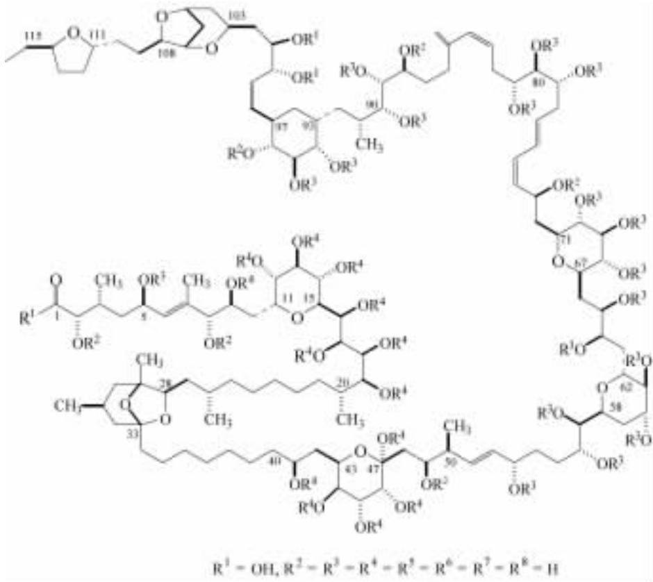
海葵毒素
