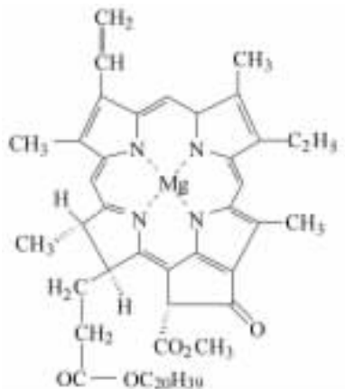
叶绿素的结构
