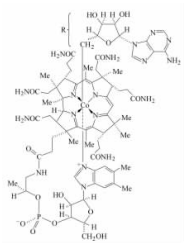
维生素 B 12
