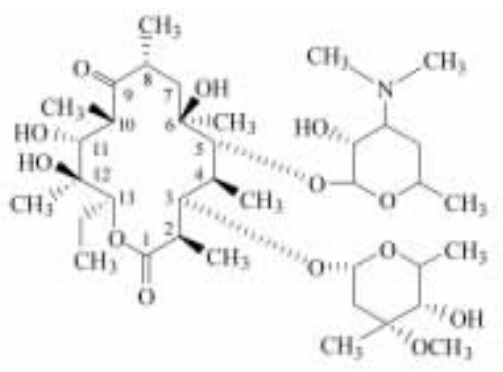
红霉素
