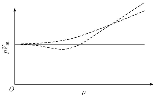
图 1-1 恒温下气体的 pV_m-p 的关系
