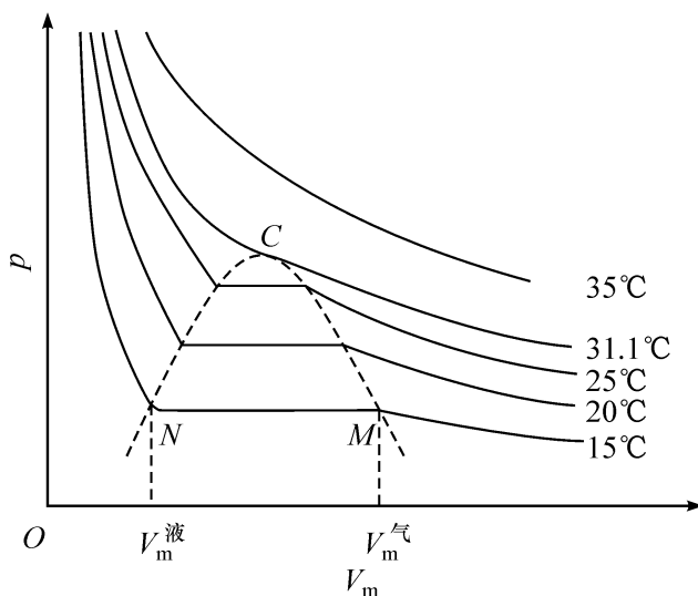
图 1-3 \text{CO}_2 液化过程
