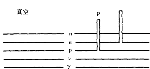
图1.1-4 根据场论给出的真空和粒子基本物理图象
