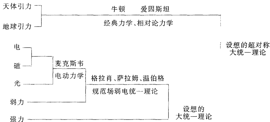
图 1.1-6 物理理论的发展趋向统一
