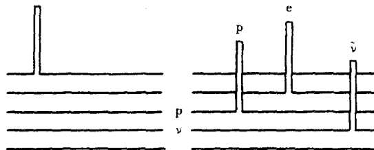
图1.1-5 中子衰变过程的场论图象
