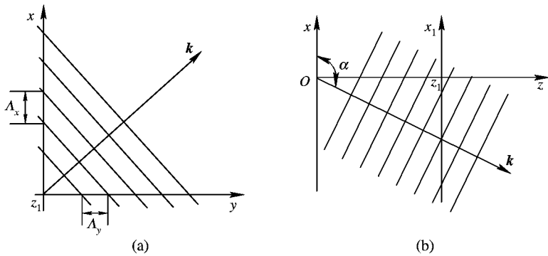
图 1.1-5 平面波的空间频率示意图 (a) k 为任意方向；(b) 空间频率分量 \xi < 0
