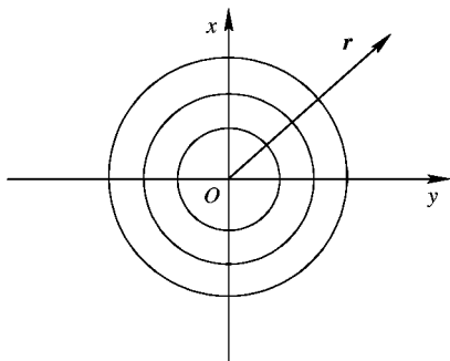
图 1.1-2 球面波示意图
