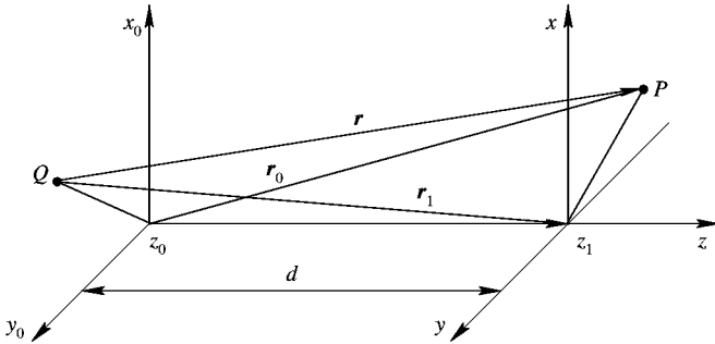
图 1.1-4 离轴发散球面波分析
