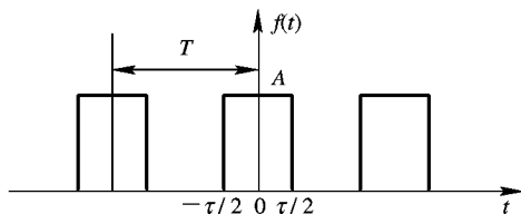
图 1.2-1 周期性矩形脉冲
