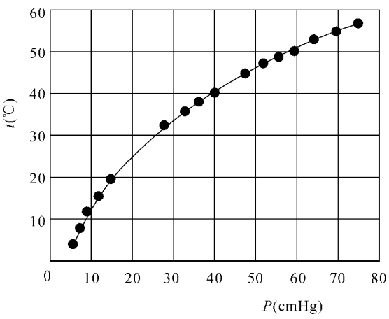
图 1 丙酮在不同温度下的饱和蒸气压图 图 2 丙酮在不同压力下的沸点
