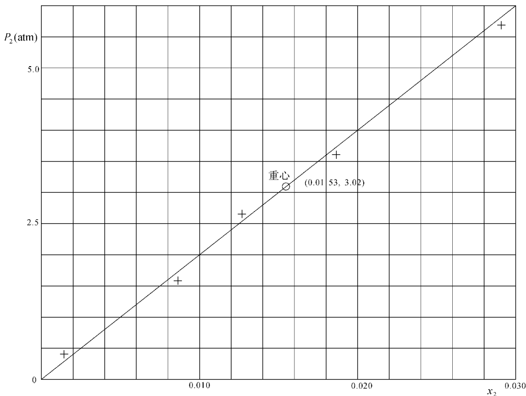
图 1-1 甲烷在戊烷中的分蒸气压
