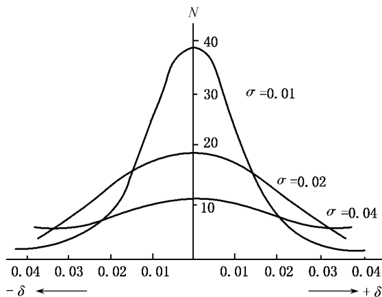
图 园 阿 疑 偶然误差正态分布曲线
