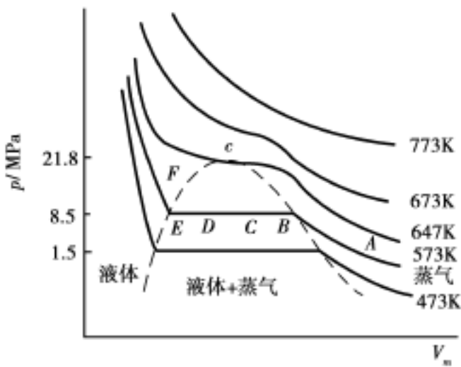
图 1-3 H 2 O 的等温线
