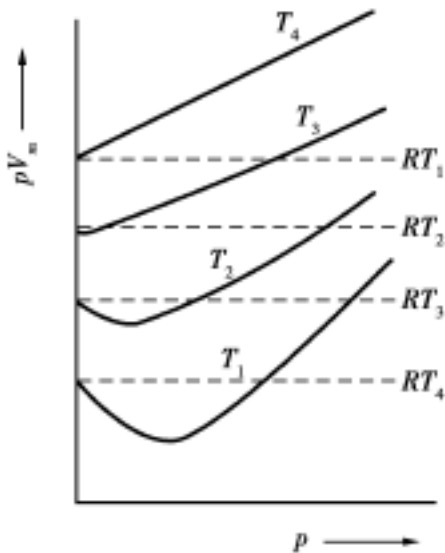
图 1-2 同一气体不同温度下的 pV_m-p 等温线
