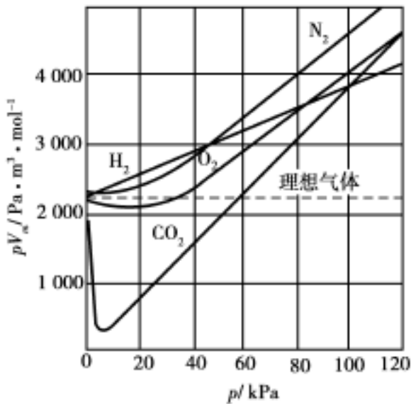
图 1-1 几种气体在 273.15K 时的 pV_m-p 等温线
