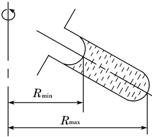
图 2-1 离心机的工作原理 注:图 2-1 引自仪器说明书、参考文献[4]
