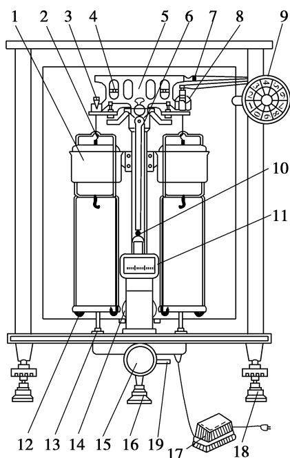
1. 空气阻尼器 2. 挂钩 3. 吊耳 4. 零点调节螺丝 5. 横梁 6. 天平柱 7. 圈码钩 8. 圈码 9. 加圈码 10. 指针 11. 投影屏 12. 称盘 13. 盘托 14. 光源 15. 旋钮 16. 底垫 17. 变压器 18. 调水平螺丝 19. 调零杆
