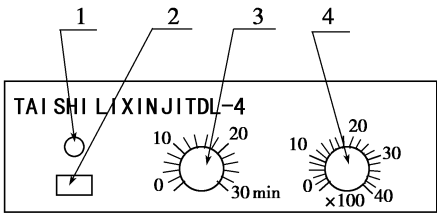
图 2-3 TDL-4 型低速台式离心机面板示意图
