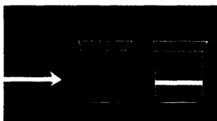
图 1-6 丁铎尔现象 左侧烧杯里是溶液，右侧烧杯里是胶体
