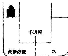
图 1-4 渗透压示意图
