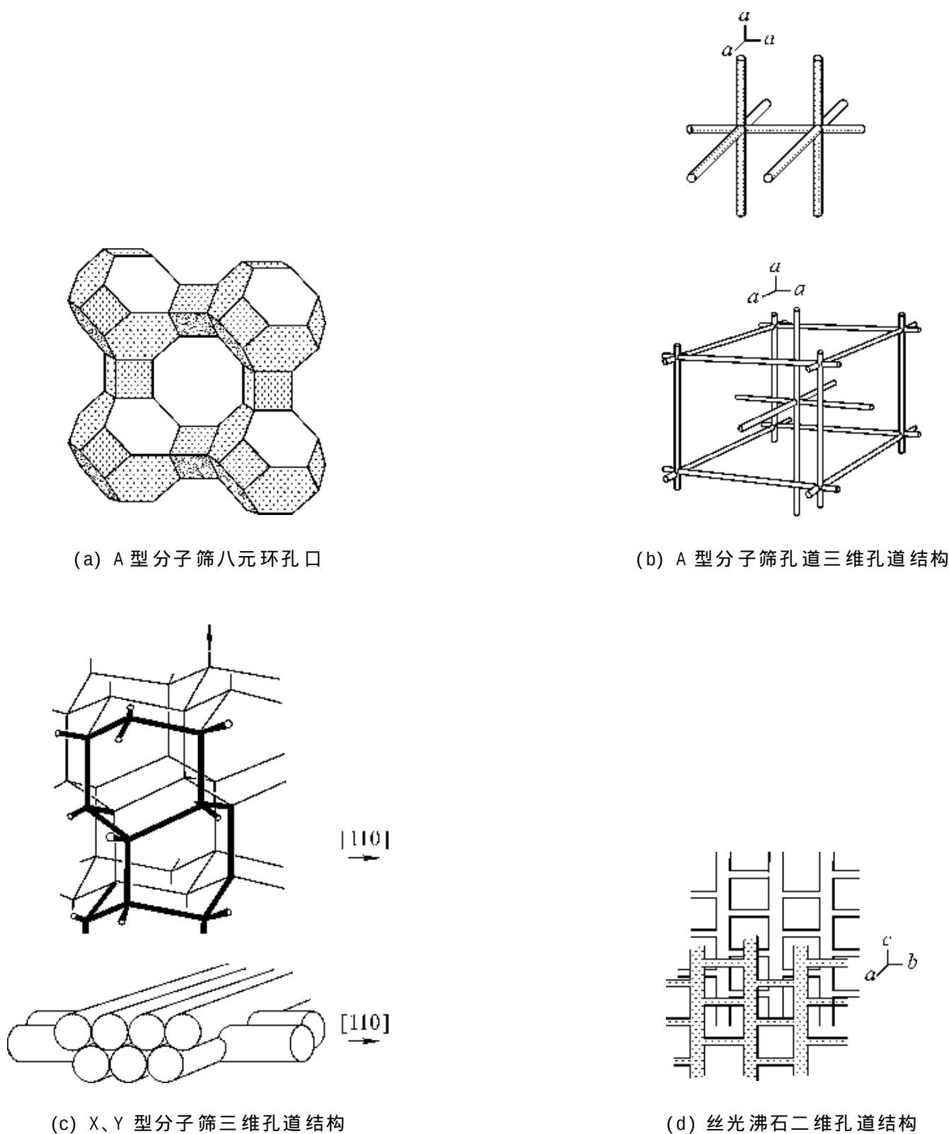
图 1 - 1 沸石分子筛结构
