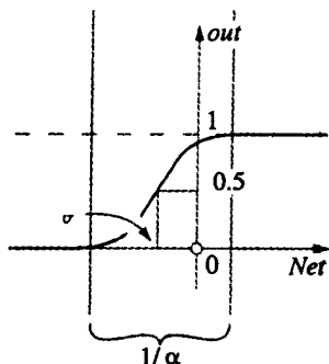
图 2-15 S 形转换函数
