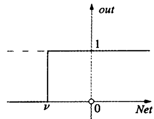
图 2-11 一个二元硬限幅器 hl(Net)
