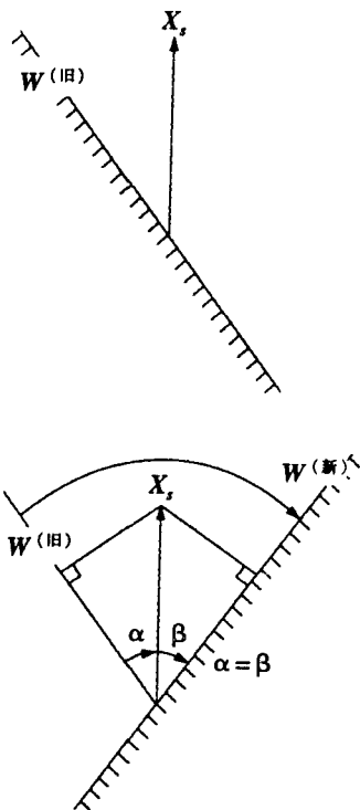
图 2-9 向量 W^{(新)} 是向量 W^{(旧)} 的镜像) 正确地将样本 X 归入另一个类中
