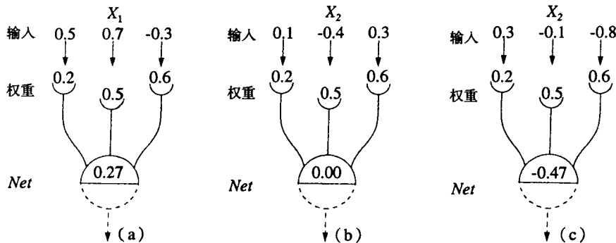
图 2-6 权重向量 W = (0.2, 0.5, 0.6) 和 3 个任意挑选的输入向量 X_1, X_2 和 X_3 之间的点积 Net
