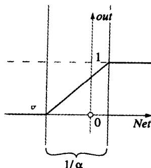
图 2-14 一个转换函数的阈值逻辑；输入量函数的线性响应宽度与 \vartheta/\alpha 成比例。交换区间起点为 -\vartheta
