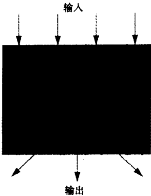
图 1-1 黑箱
