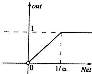
图 2-13 阈值逻辑
