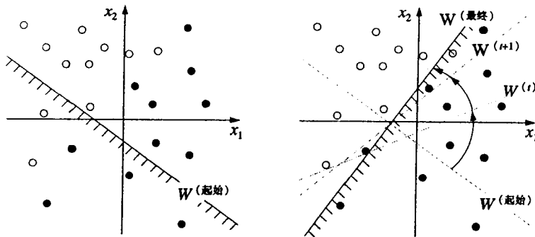
图 2-7 将判定向量 W 朝着更好的位置改变： W^{(t+1)} 是一个比 W^{(t)} 更好的判定向量，因为 W^{(t+1)} 分类时仅有两个样本失败；而 W^{(t)} 则有 5 个样本失败。理想判定向量 W 将全部 C_1 类的样本与全部 C_2 类样本（圆圈）分开。
