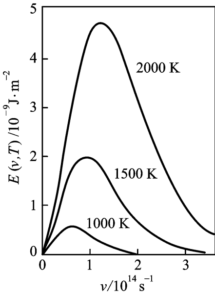
图 1.1 黑体辐射分布曲线
