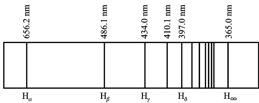
图 1.2 氢原子在可见和近紫外区域的发射光谱
