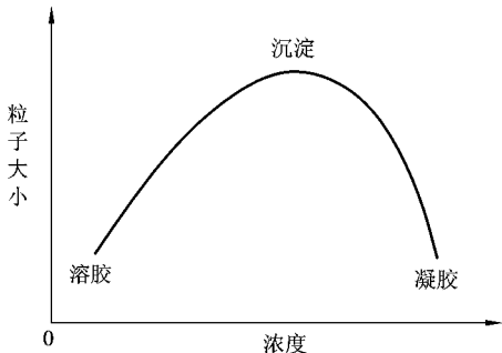
图 员- 员 颗粒大小与反应物浓度的关系
