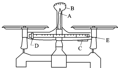
图 猿- 员 摇台天平
