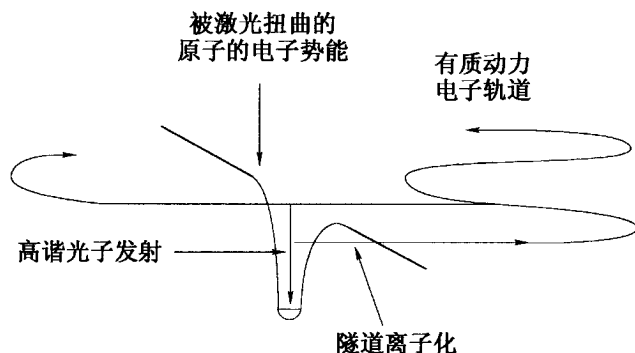
图 1.1 一束强的、超快的激光脉冲与一个原子之间相互作用之后所发生的结果。电子的势能结构，原本应该会在最小值的两侧均呈现对称状态，从而将电子限制在原子核的邻近区域，现在却被激光辐射所扭曲。电子首先离子化，从原子中释放出来，而后沿着由它的有质动能决定的、在激光脉冲的电场中形成的振动轨道通过隧道化越过处于低势能的能障。如果电子的轨道能将其带回到离子化的原子的核周围，由于带负电的电子被带正电的离子所加速，就会发生高频光子的发射。现已发现，这个高频光子是与最初被原子吸收的激光频率完全谐调的谐波。
