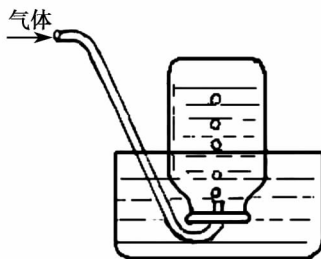
图 1-6 排水集气法
