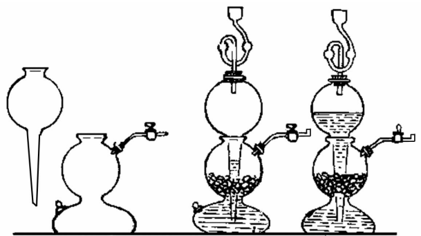
图 1-1 实验室常用的启普发生器的构造图
