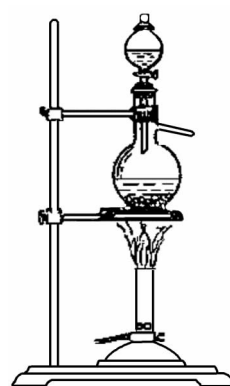
图 1-2 实验室常用的发生气体的装置
