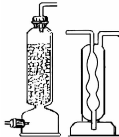
图 1-4 干燥塔
