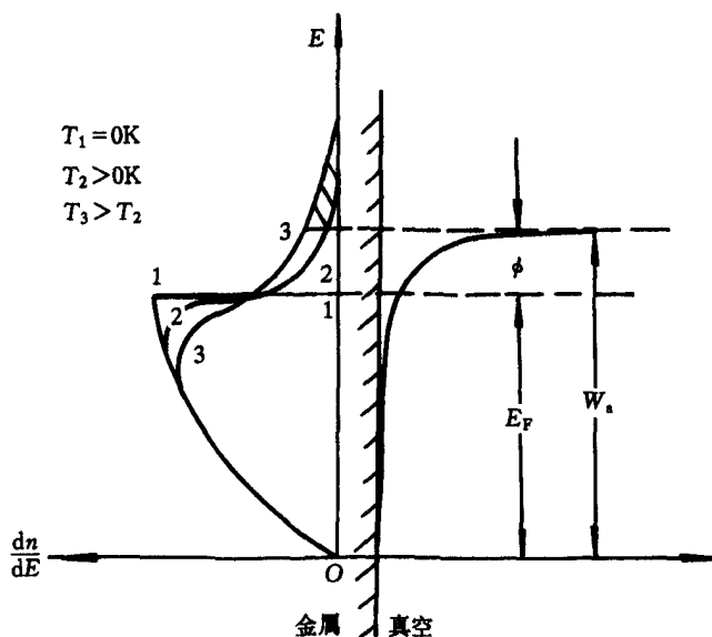
图 1.3.1 金属的表面势垒和内部电子的能量分布
