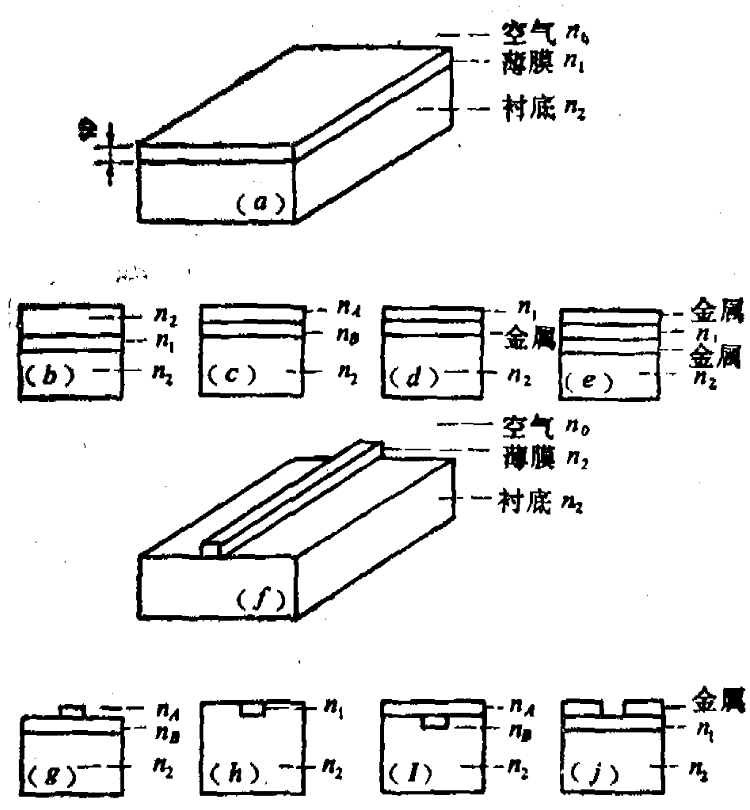
图1-1-1 各种光波导
