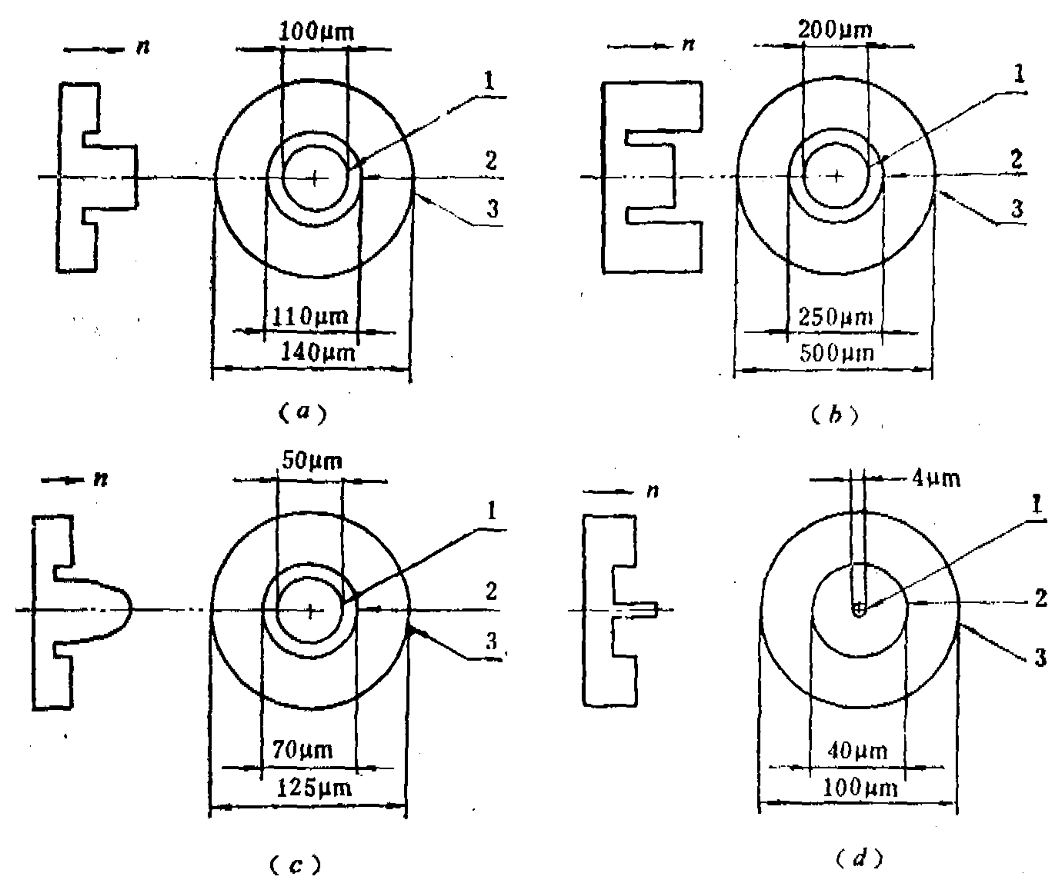
图1-1-2 某些光纤的典型尺寸和折射率分布(1-芯, 2-芯区与包层区间的过渡层, 可以没有, 3-包层) (a)多模阶跃折射率光纤; (b)塑料包层多模光纤; (c)多模渐变折射率光纤; (d)单模阶跃折射率光纤
