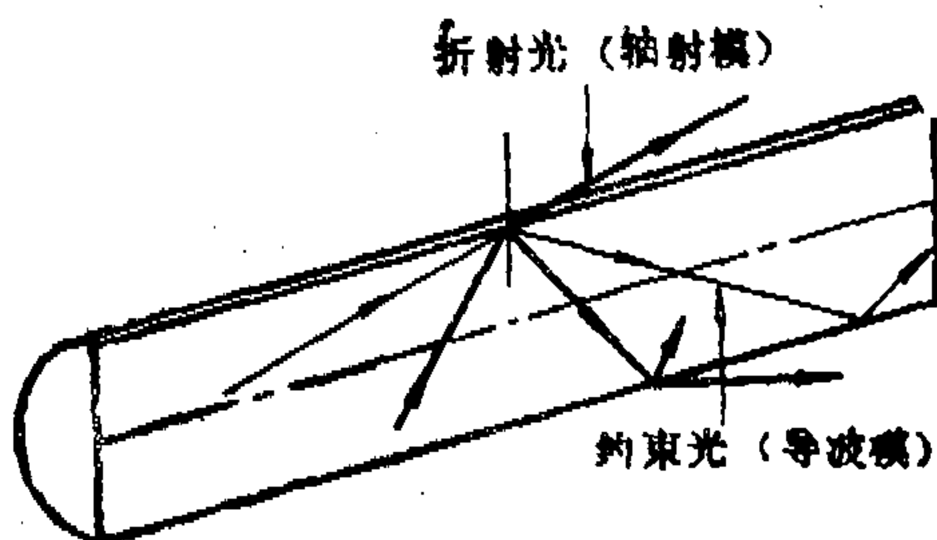
图1-1-3 约束光(导波模)和折射光(辐射模)
