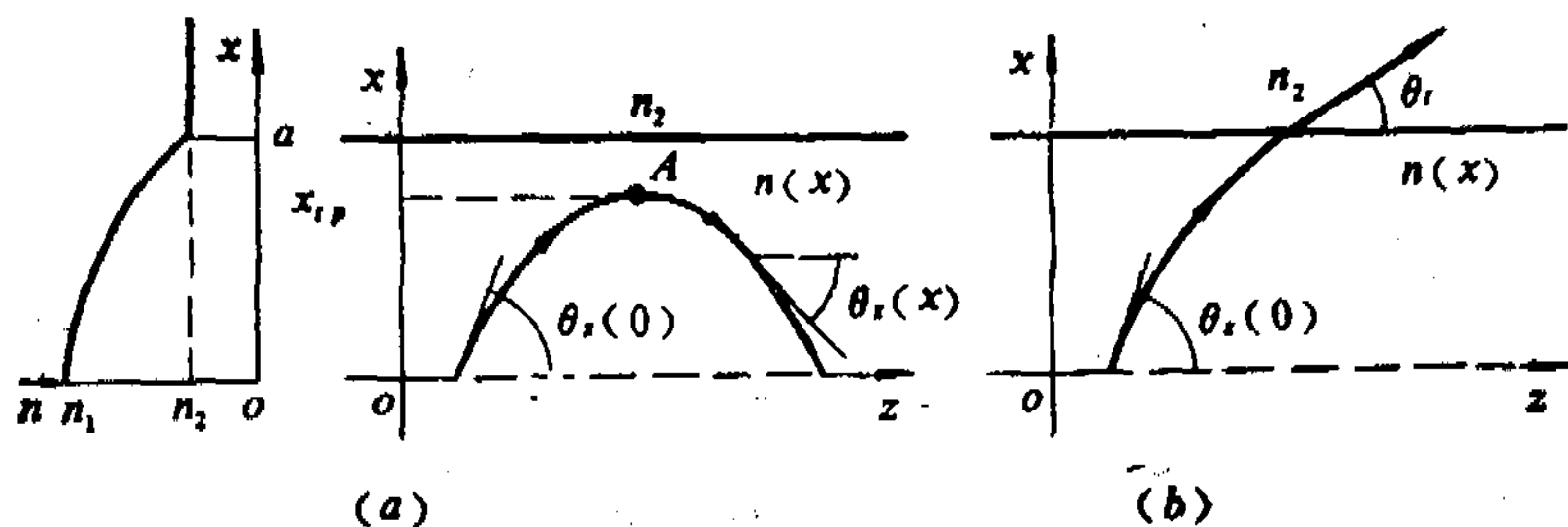
图1-2-3 一维限制渐变光波导中的光线
