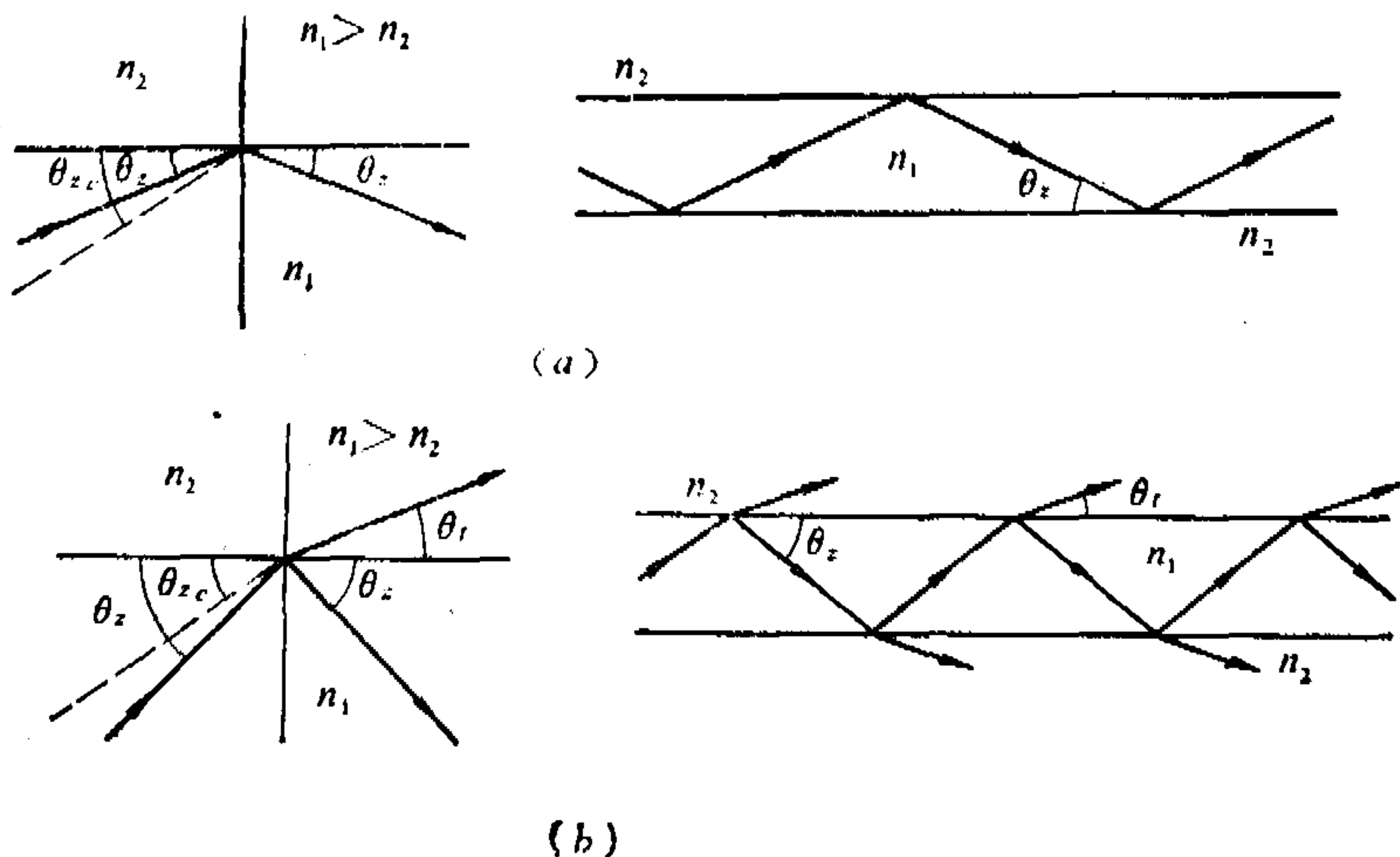
图1-2-2 一维限制阶跃光波导中的光线
