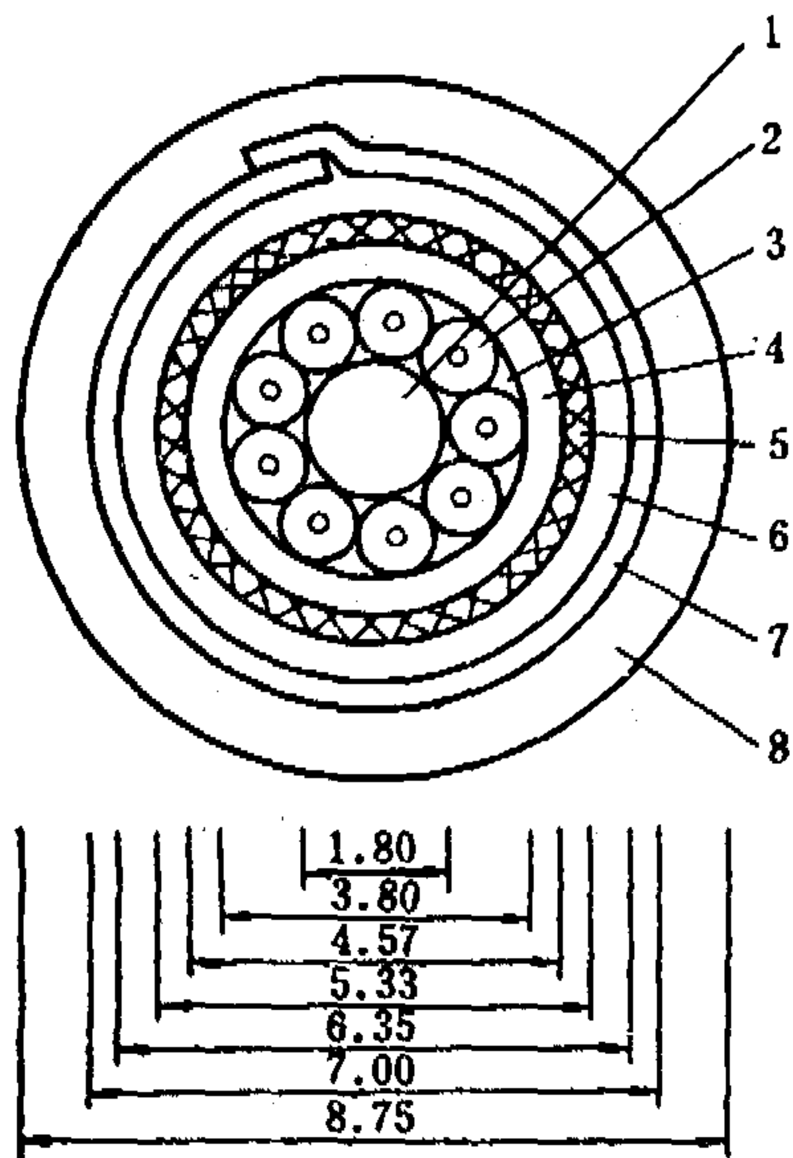
图1-5 九芯光缆结构及尺寸示意
