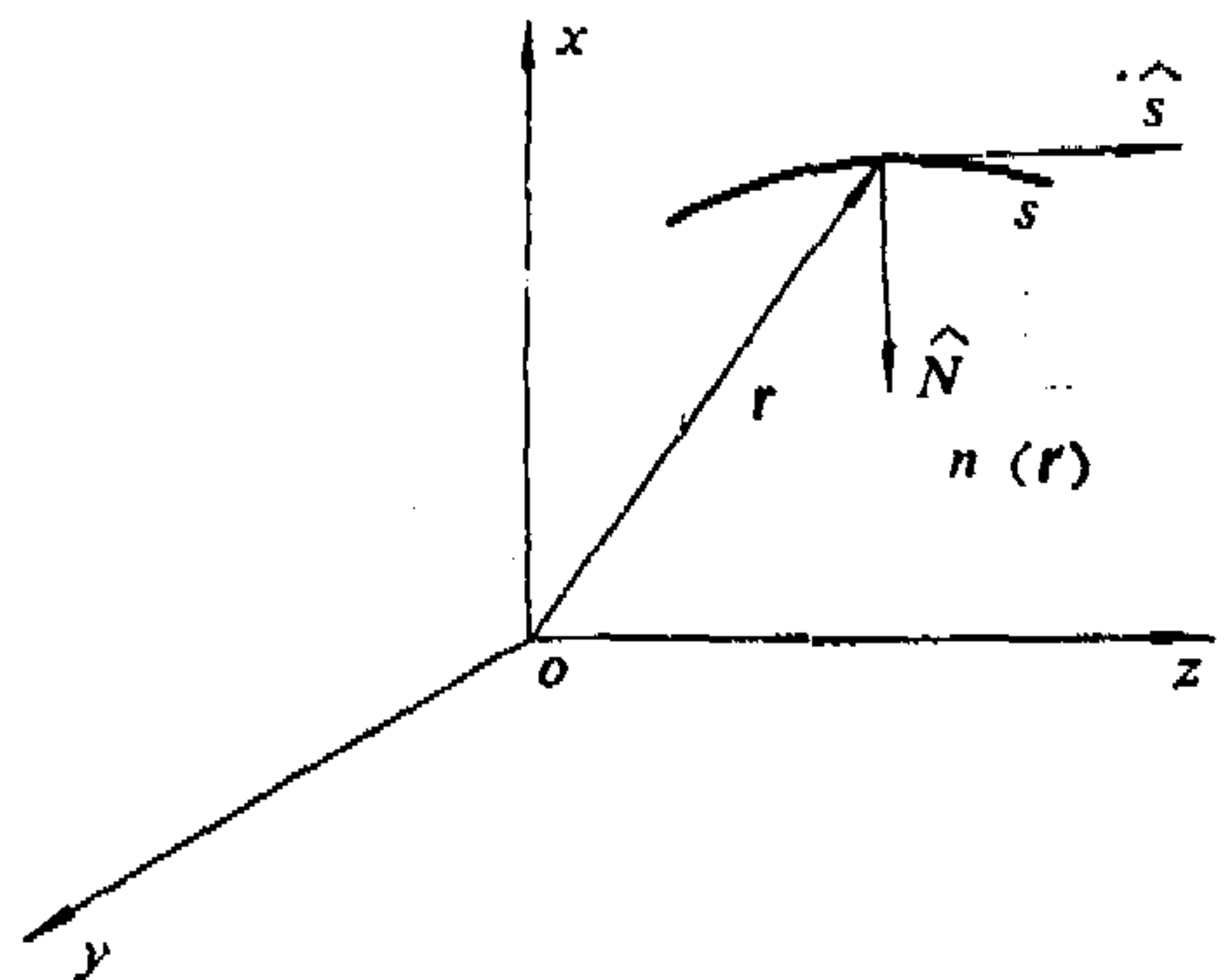
图1-2-1 光线轨迹
