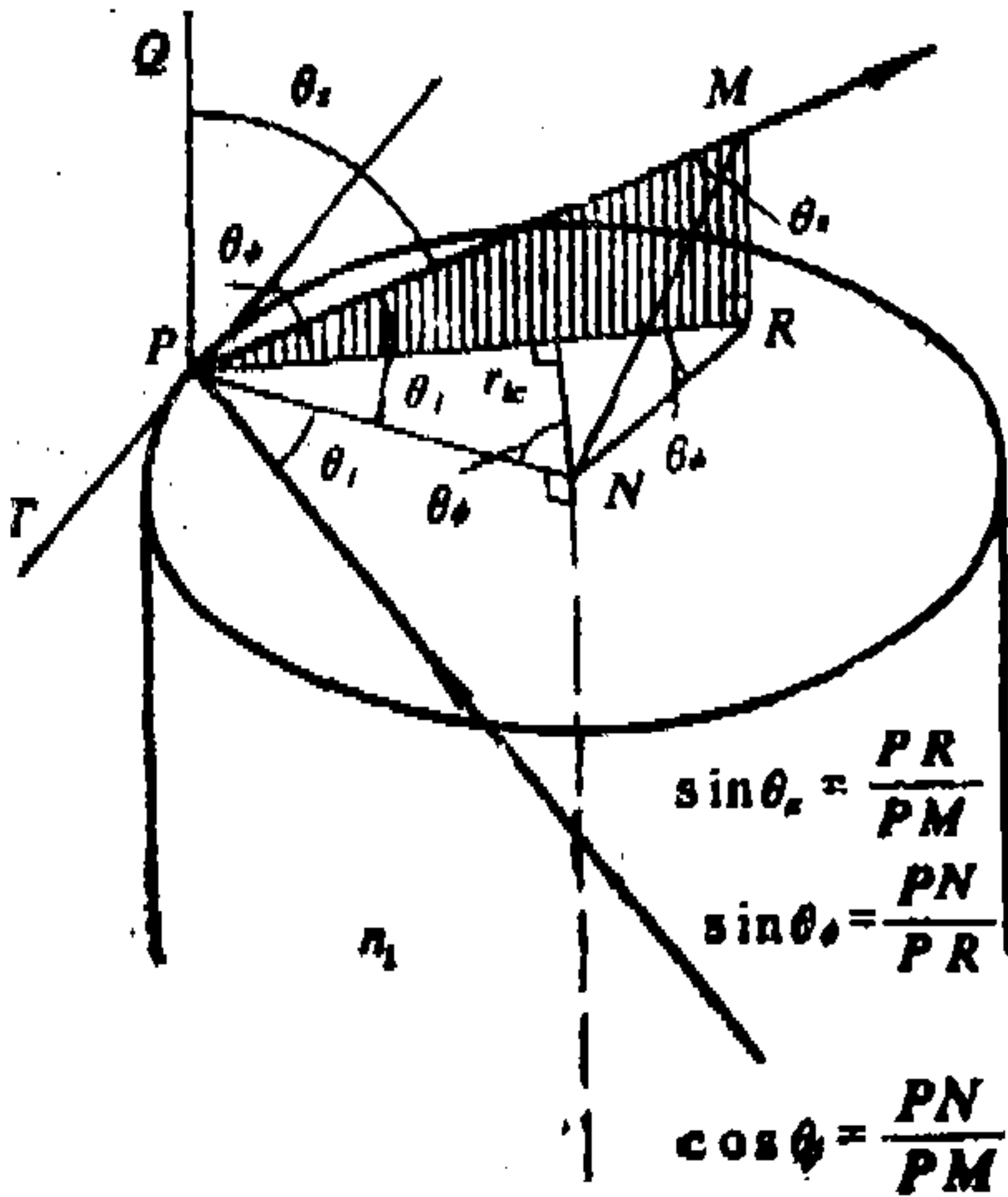
图1-2-6 阶跃光纤界面处的入射光与反射光
