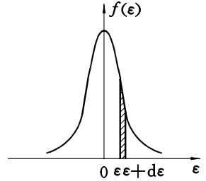
图园-员 高斯正态分布曲线
