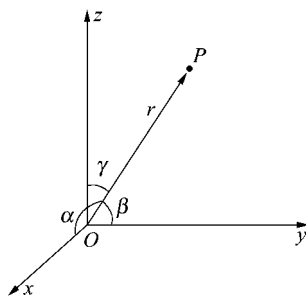
图 1.3-1 位矢
