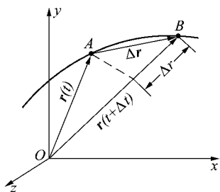
图 1.3-2 位移
