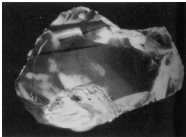
图 1.4 金刚石晶体在阴极射线中发光 [3]
