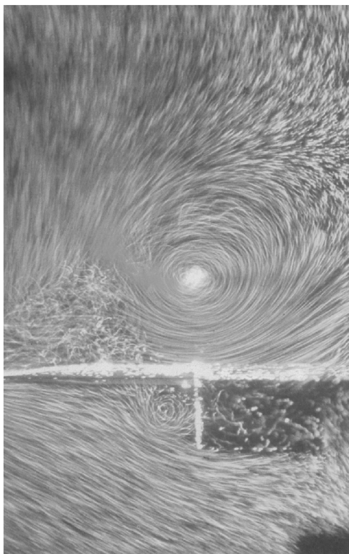
图 1.6 超声气流在飞行体附近形成的涡旋 [3]
