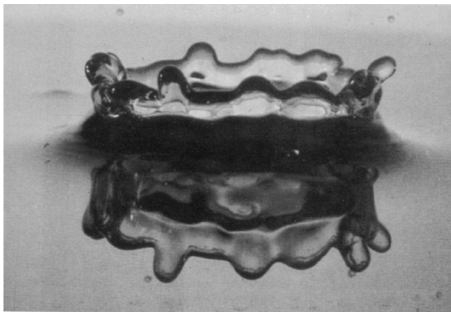
图 1.5 液滴落在液面上的一瞬间 [3]
