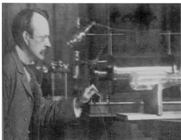
图 1.3 汤姆逊发现电子 [3]
