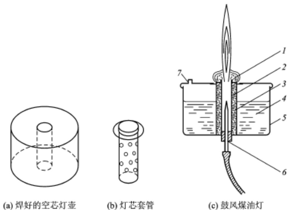
图 2-1 煤油喷灯的构造
