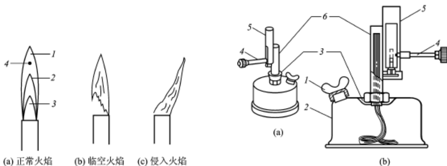
图 2-2 正常火焰与不正常火焰
