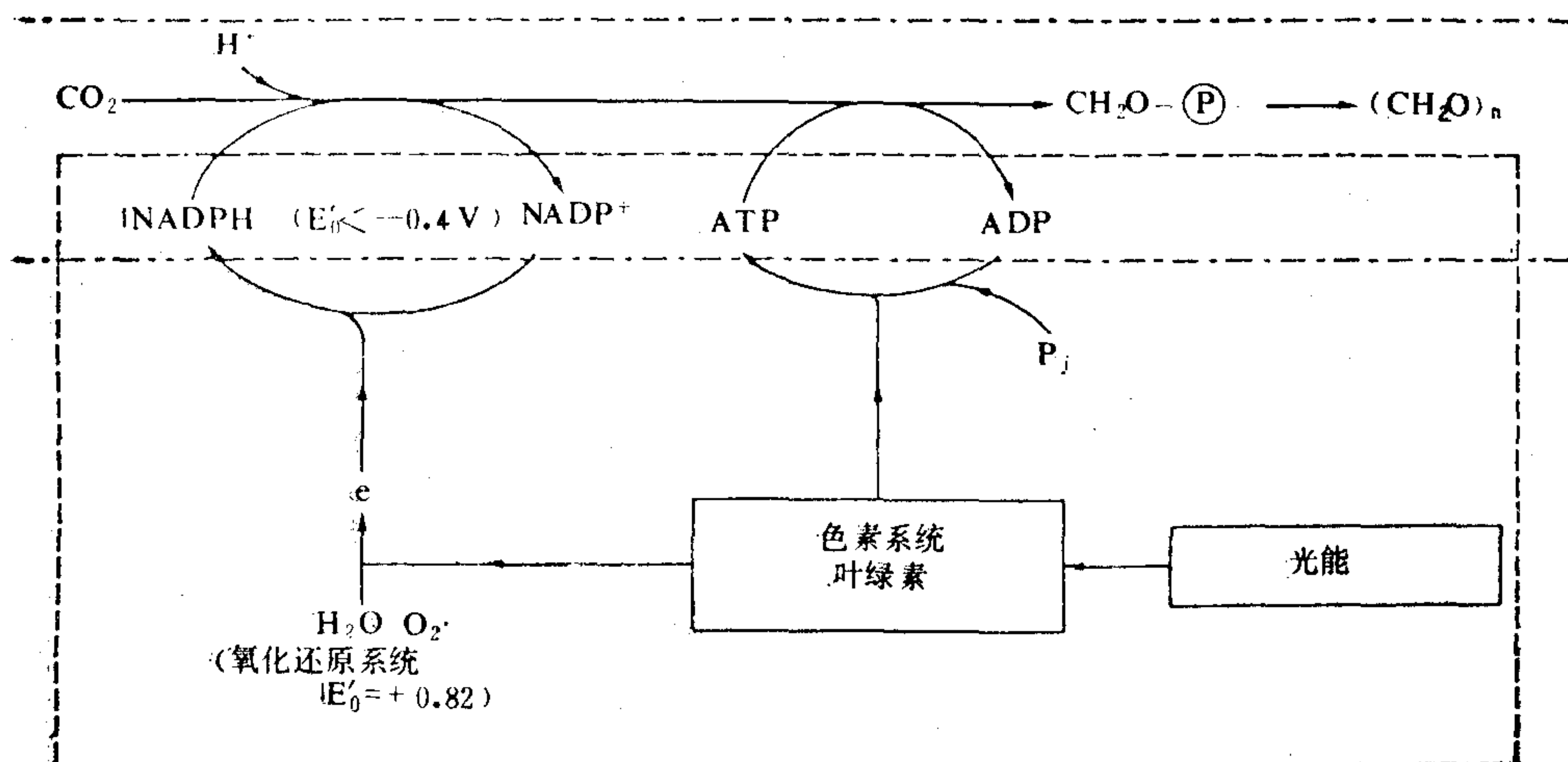
图 2—1 光合作用简要过程 - · - · - · - 暗阶段 - - - - - 光阶段
