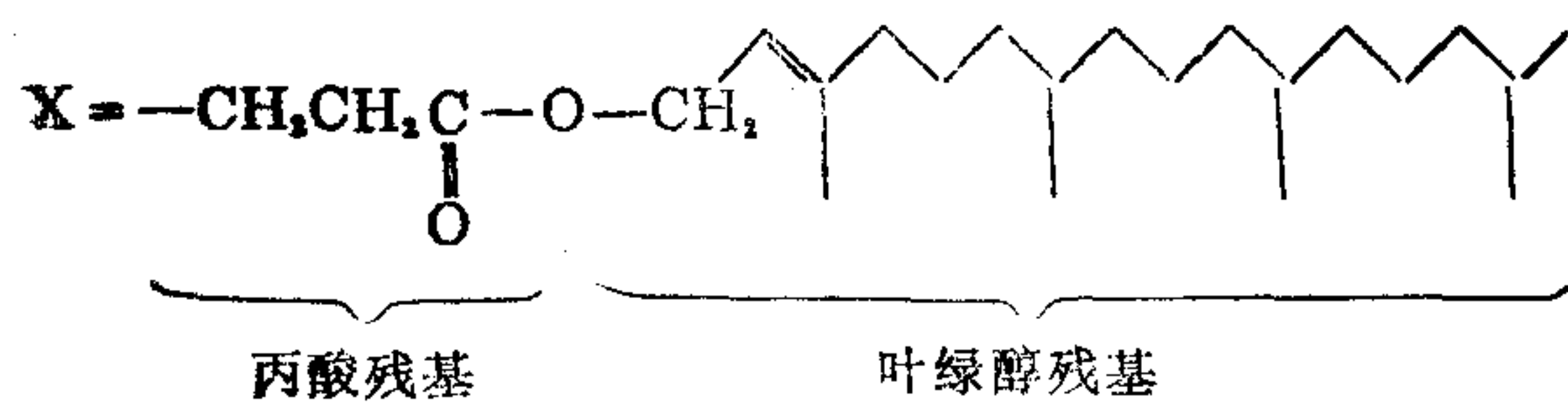
图 2—3 叶绿素结构式
