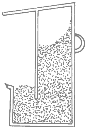
图 6 自动式食槽
